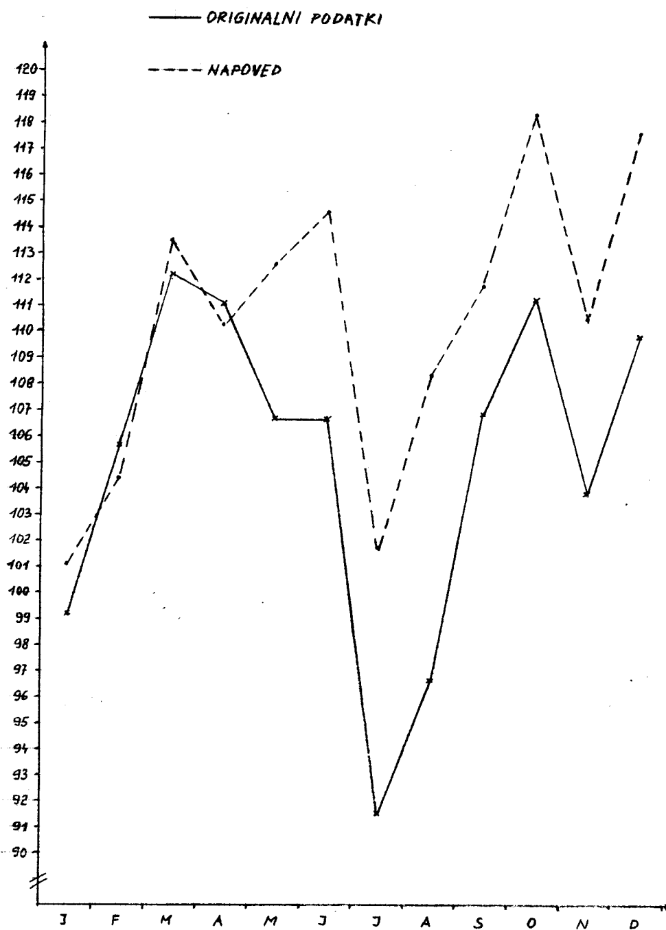
SLIKA 5: INDEKS INDUSTRIJSKE PROIZVODNJE SR SLOVENIJE V L. 1975 (100 = Ø 1974)
